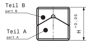
Zusammengebauter Zustand 13.7 Assembled condition 13.7
