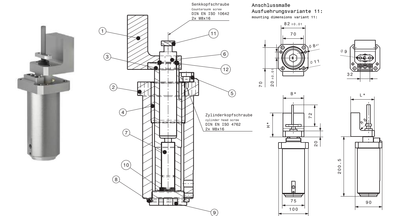
Lieferumfang Ausführung 11: Scope of delivery variant 11:
