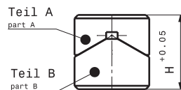
Zusammengebauter Zustand 13.6 Assembled condition 13.6
