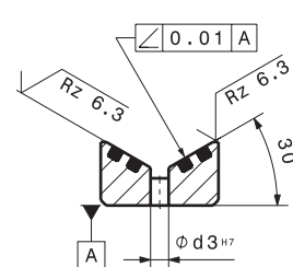
Schnitt B-B View B-B
