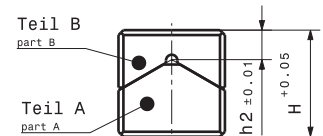
Zusammengebauter Zustand 13.7 Assembled condition 13.7
