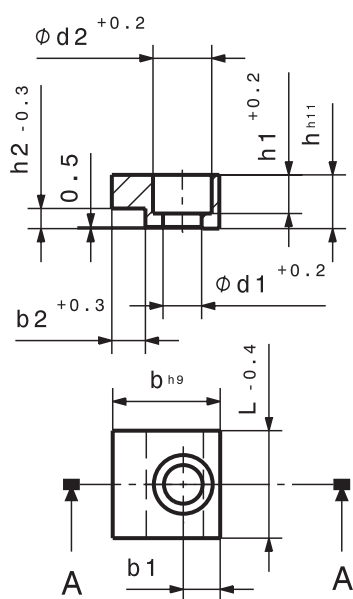
Schnitt A-A
